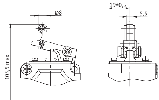
Выключатель ВПК2113
