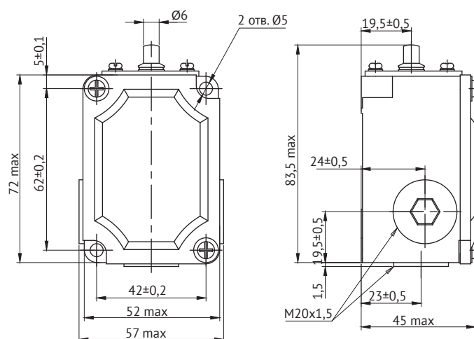
Выключатель ВПК2110
