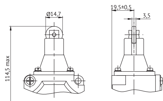
Выключатель ВПК2113
