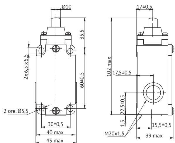
Выключатель ВП15К21А-211
