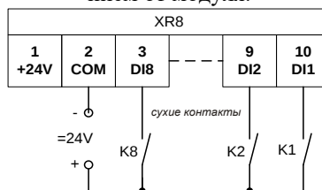
Рис.1. Вариант подключения сухих контактов с питанием от модуля.
