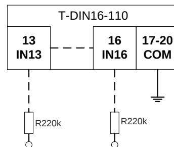
Точки контроля наличия напряжения 220 В
