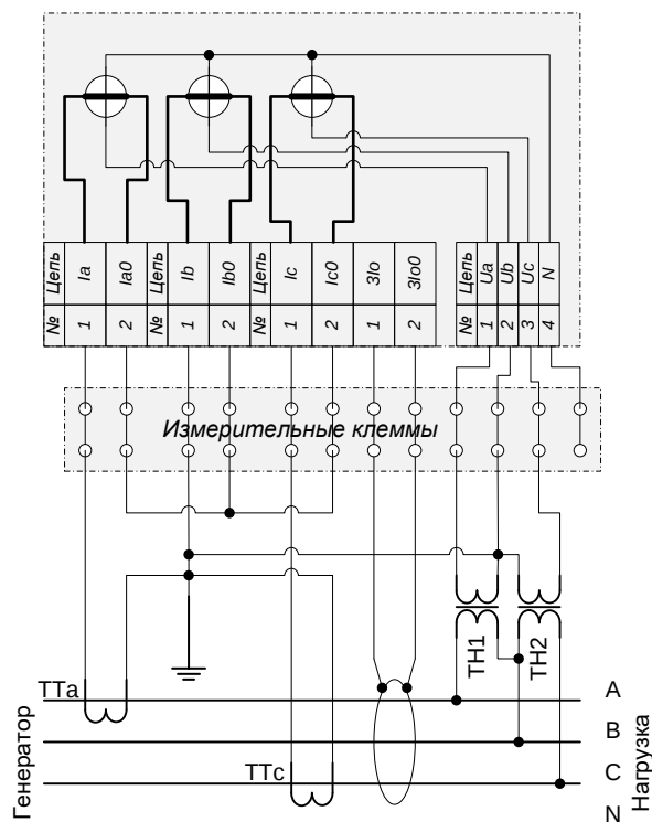
4. Схема подключения модуля к трехфазной 3-х проводной сети с помощью двух трансформаторов напряжения и двух трансформаторов тока
